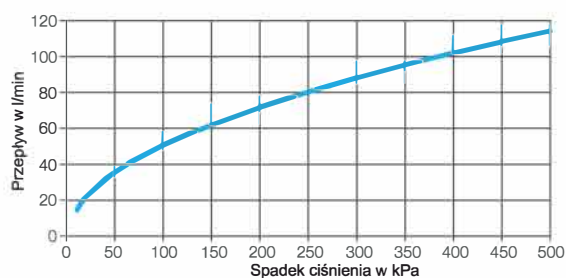
Wykres przepływu
