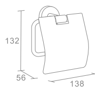
740006 Papierrollenhalter / Toilet Roll Holder
